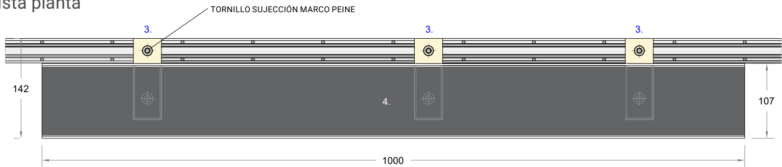
Vista planta
