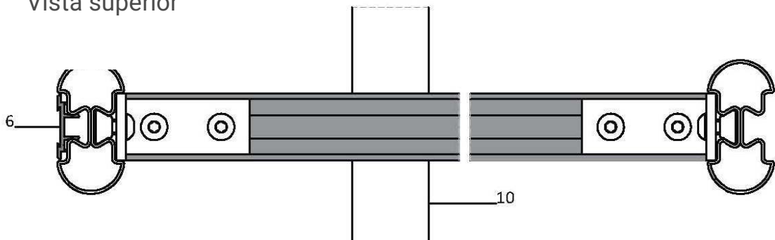
Vista superior
