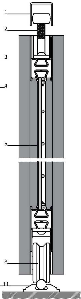
Sección frontal
