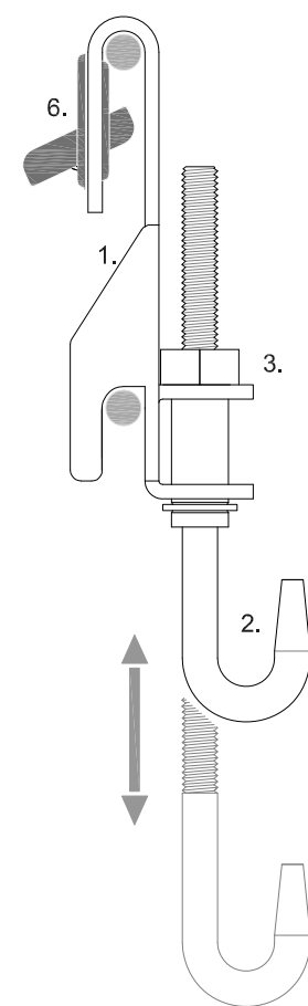
Vista lateral
