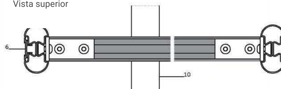
Vista superior
