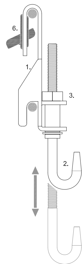
Vista lateral
